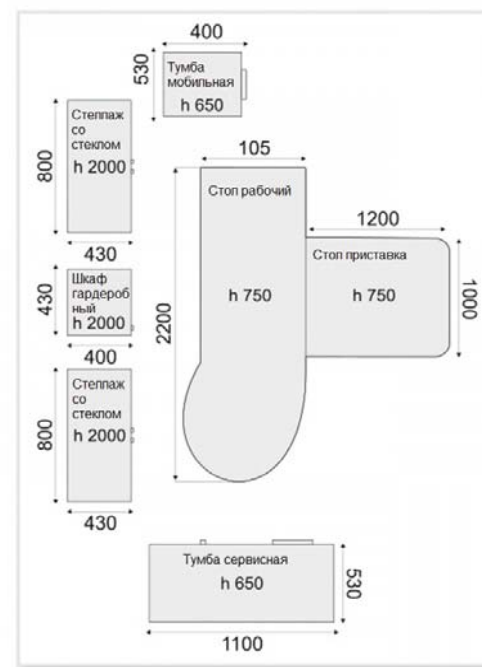
Эскиз/схема, комплекта офисной мебели (6 предметов)
