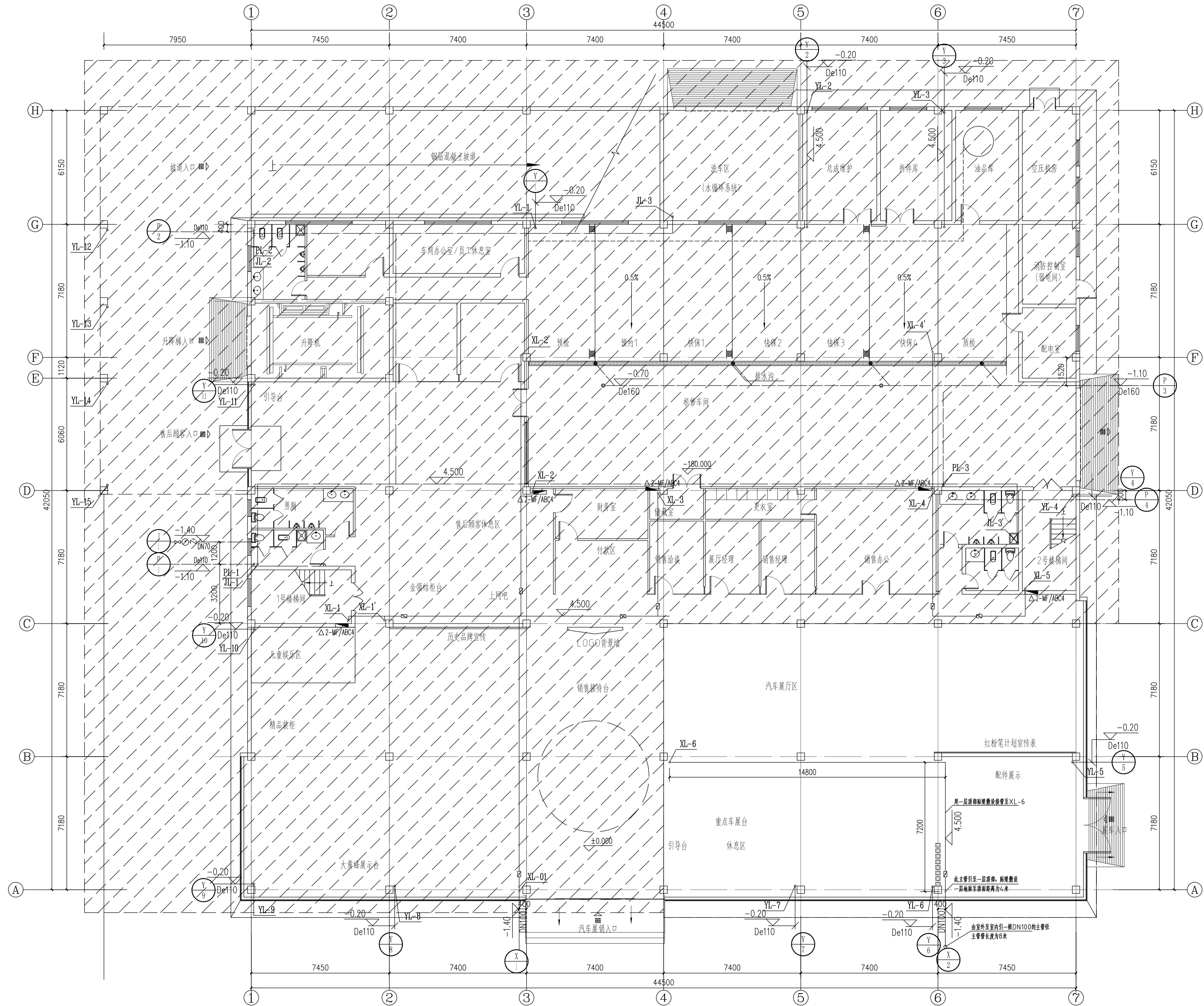
一层给排水、消防平面图 1:100
