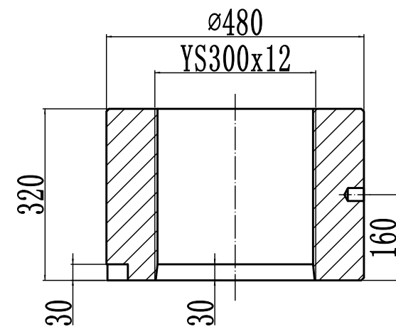
3000T主拉杆螺母, 8件, 单重0.28T
