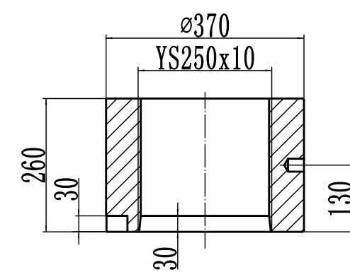
5000T拉杆螺母, 22件, 单重0.12T
