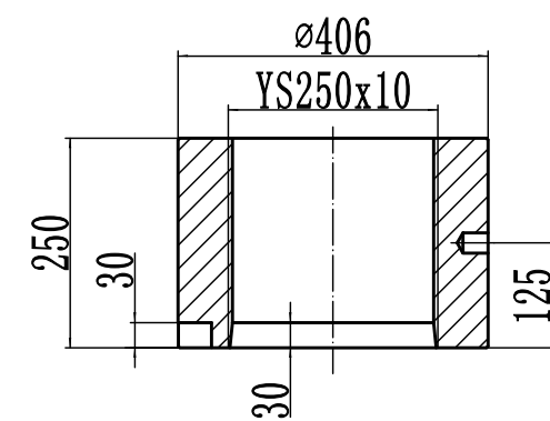
3000T副拉杆螺母, 2件, 单重0.16T
