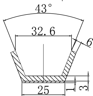
A-A 2:1
