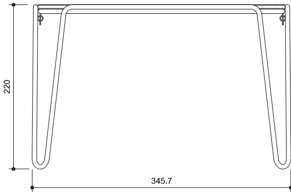
SIDE VIEW 侧视图 SCALE: 1:5
