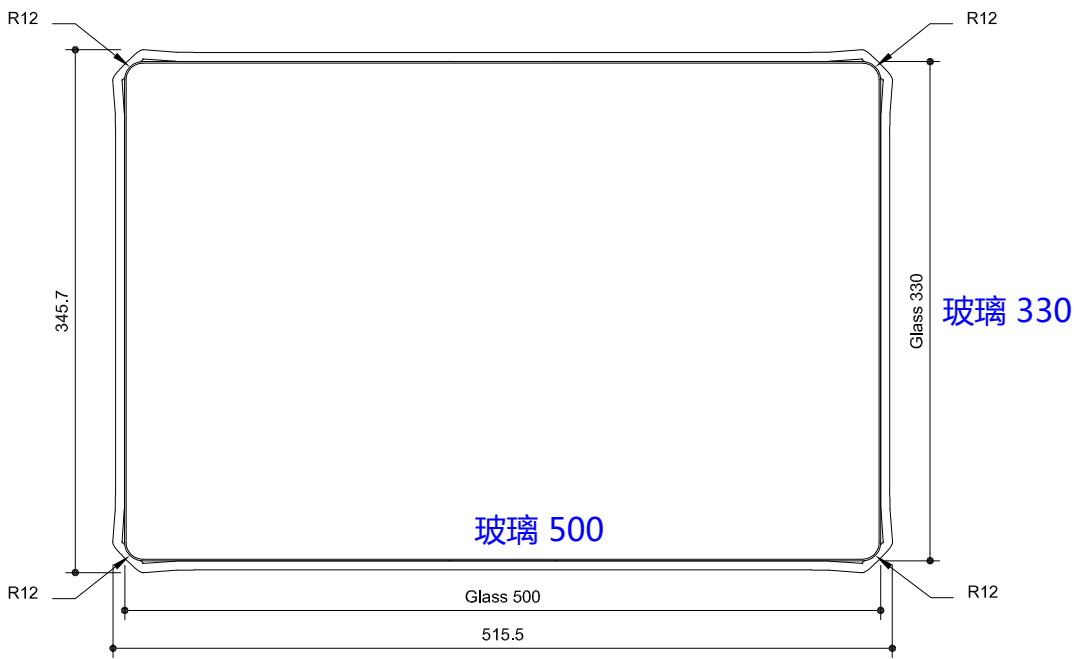
TOP VIEW 俯视图 SCALE: 1:5
