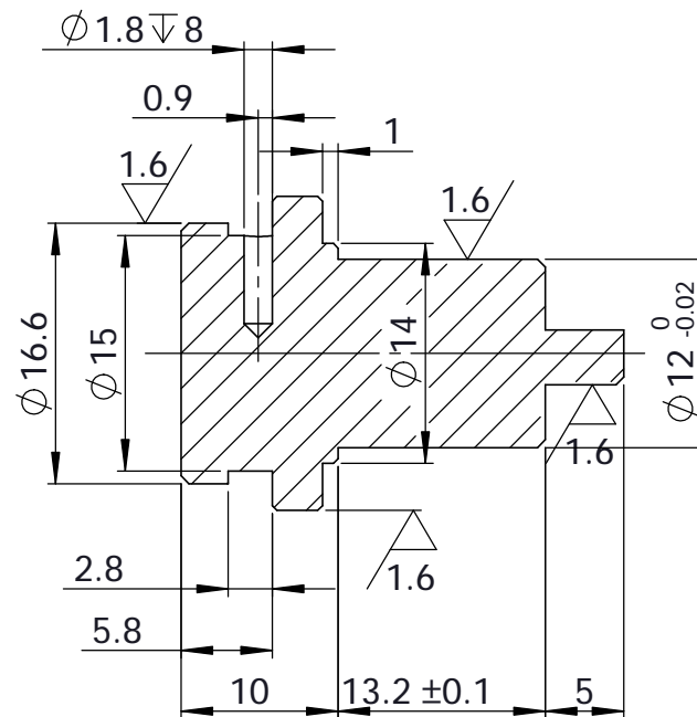
剖面 A-A
