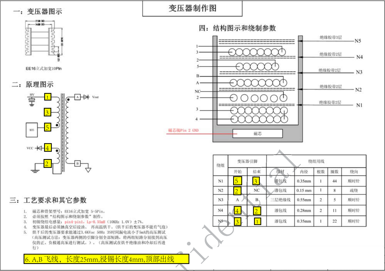
图 5 变压器制作规格书
