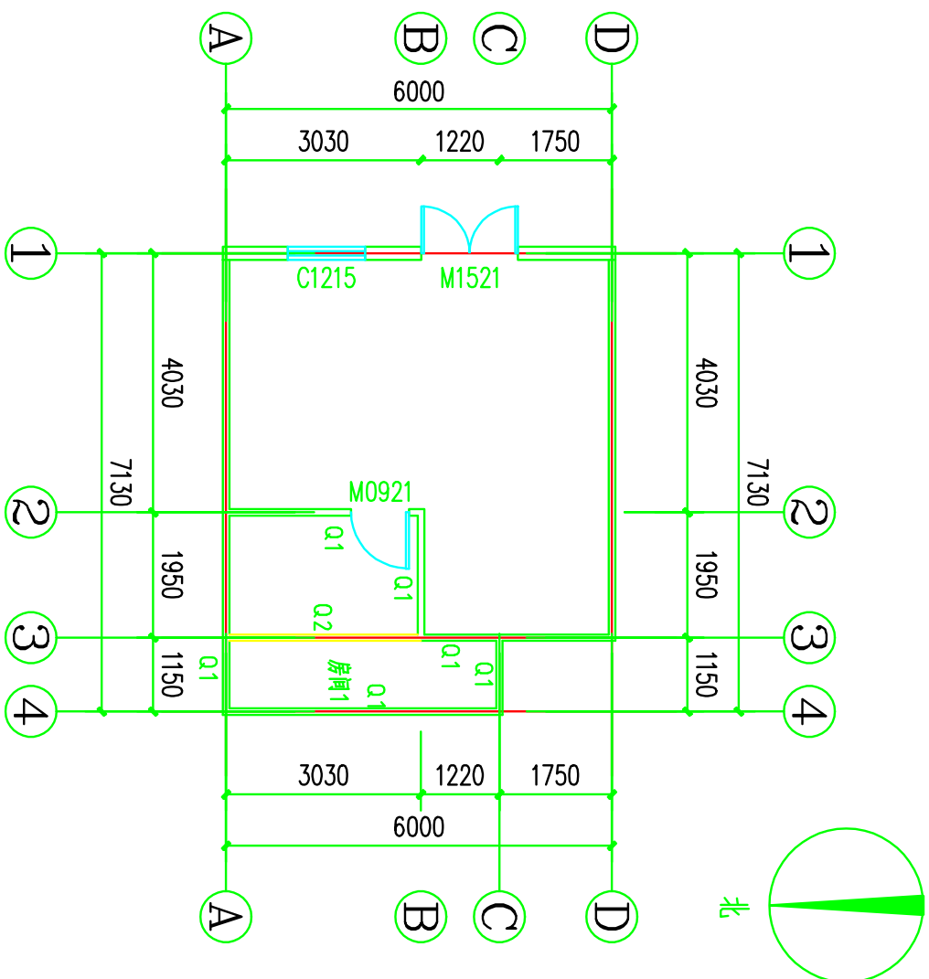
中兵北福保险房间改造平面图
