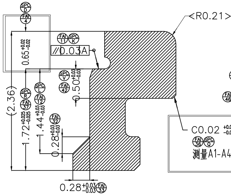
断面图 A-A 比例 25 : 1
