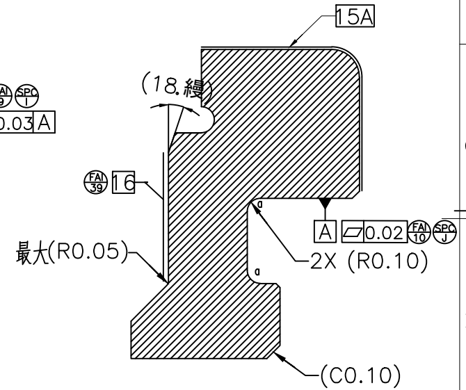
断面图 A-A 比例 25 : 1
