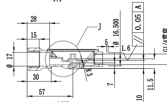
剖面 I-I 比例 1:2
