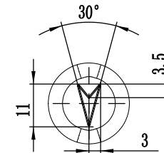
局部视图 E 比例 1:1
