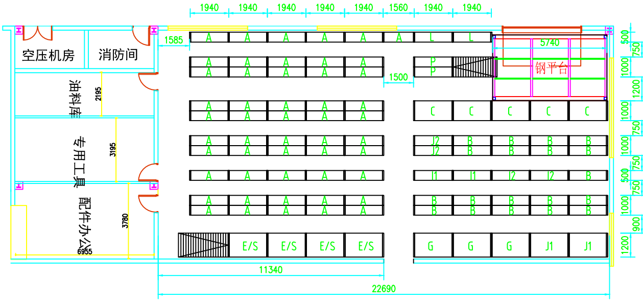
阁楼1层
