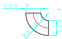
OD323.9非标直角弯头 数量 1
