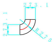
OD273.1非标直角弯头 数量 1
