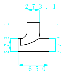
OD273.1斜三通 数量 2
