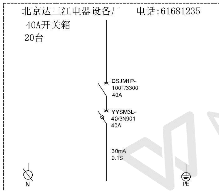
室外防雨配电箱 箱体尺寸: 350*450*230 颜色: 桔红色 支架: 800MM
