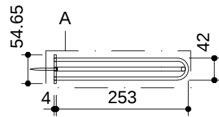
俯视图 SCALE: 1:10
