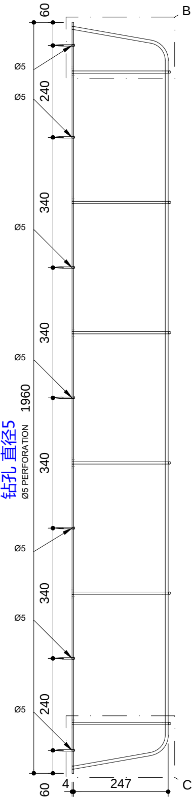
SIDE VIEW SCALE: 1:10
