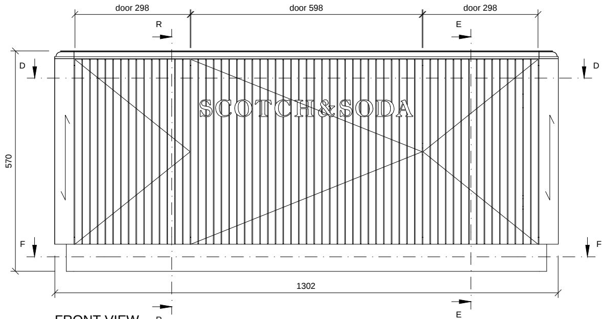
FRONT VIEW SCALE 1:10 正面图
