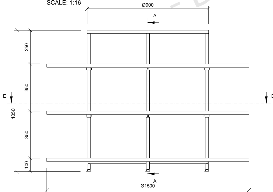
正面图 FRONT VIEW SCALE: 1:16
