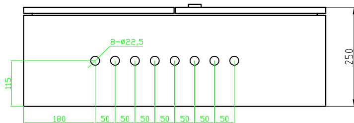
主视图
