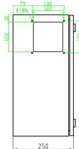
左视图
