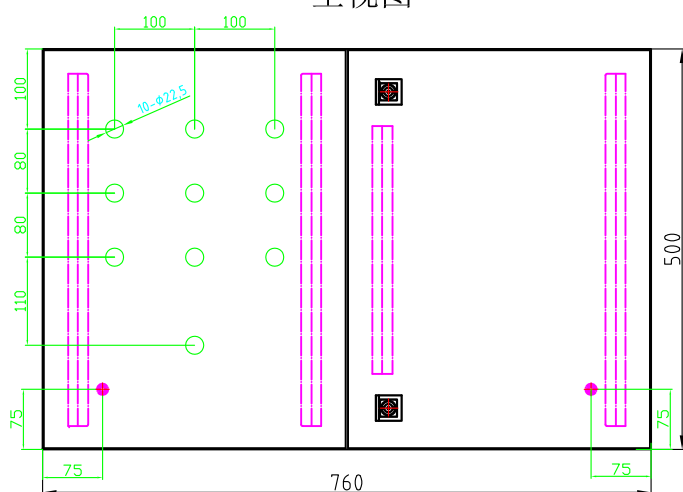
主视图
