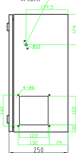
右视图
