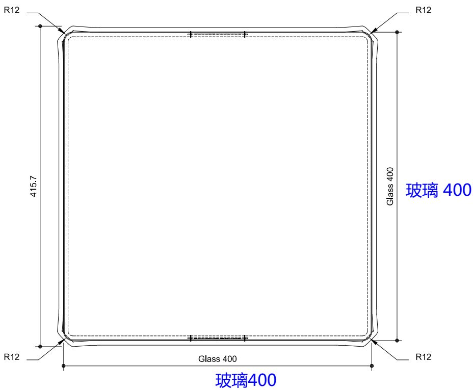
TOP VIEW SCALE: 1:5 俯视图
