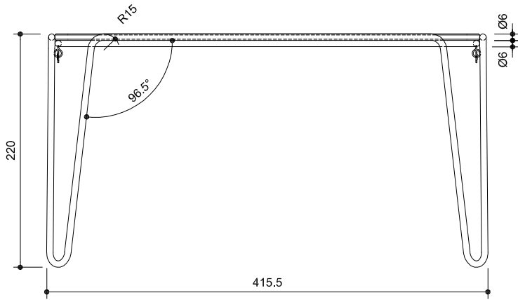
SIDE VIEW SCALE: 1:5 侧视图
