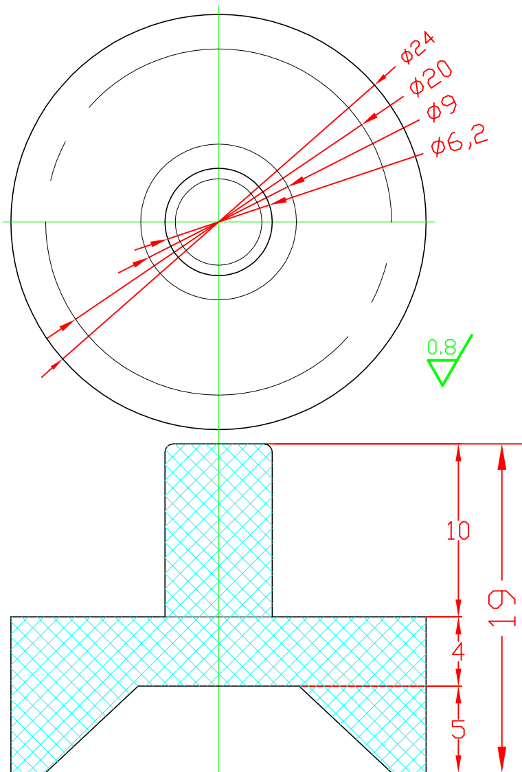
脚垫1：气相硅胶制造，硬度50
