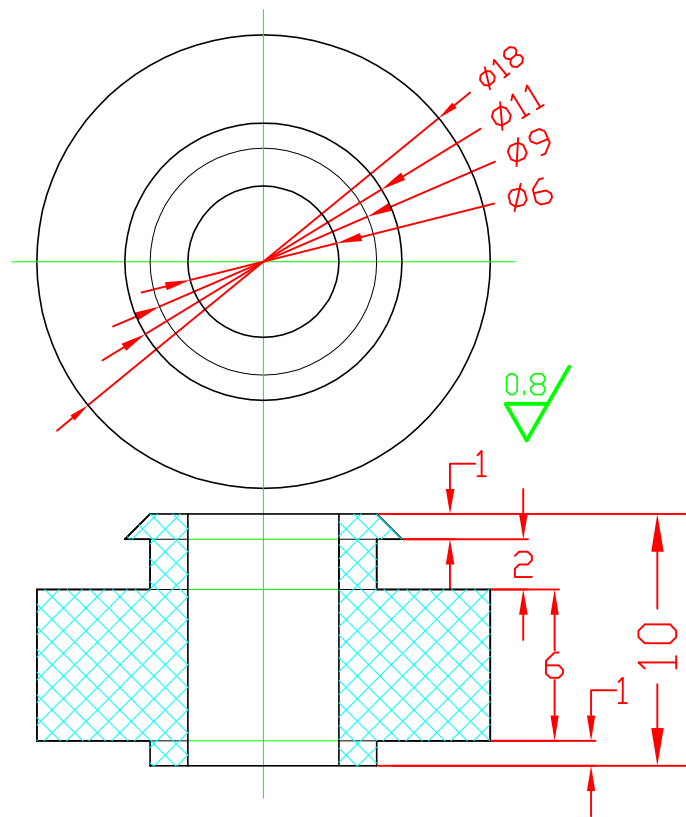
脚垫2：气相硅胶制造，硬度50
