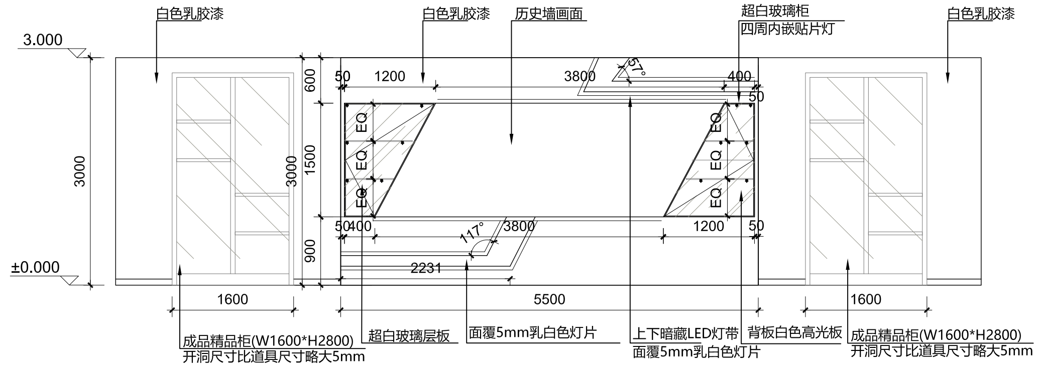
精品柜/品牌历史抢墙立面图 ELEVATION SCALE 1:50
