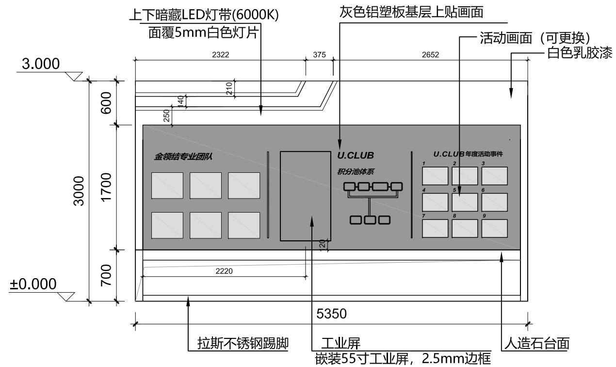
水吧台立面图 ELEVATION SCALE 1:50
