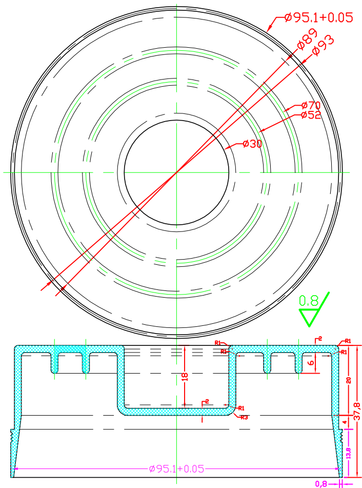
收料碗：高质量气相硅胶制造，硬度68
