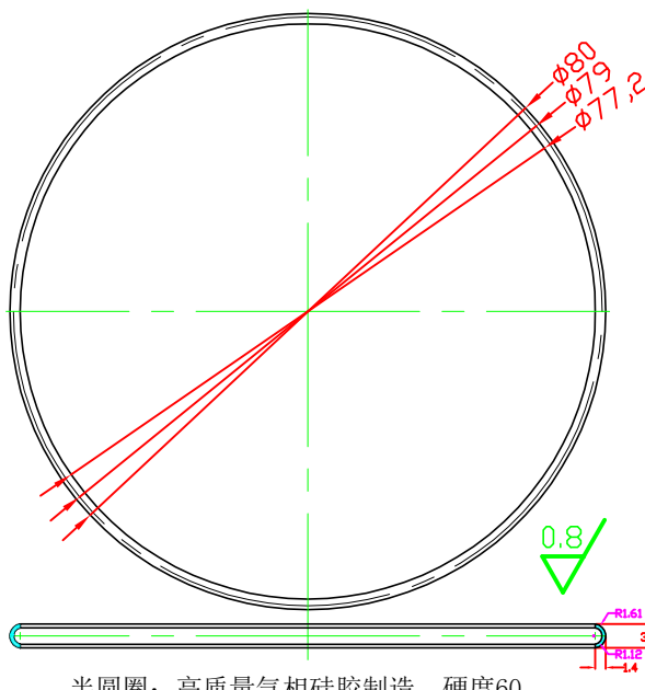
半圆圈：高质量气相硅胶制造，硬度60
