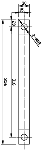
管箍详图
